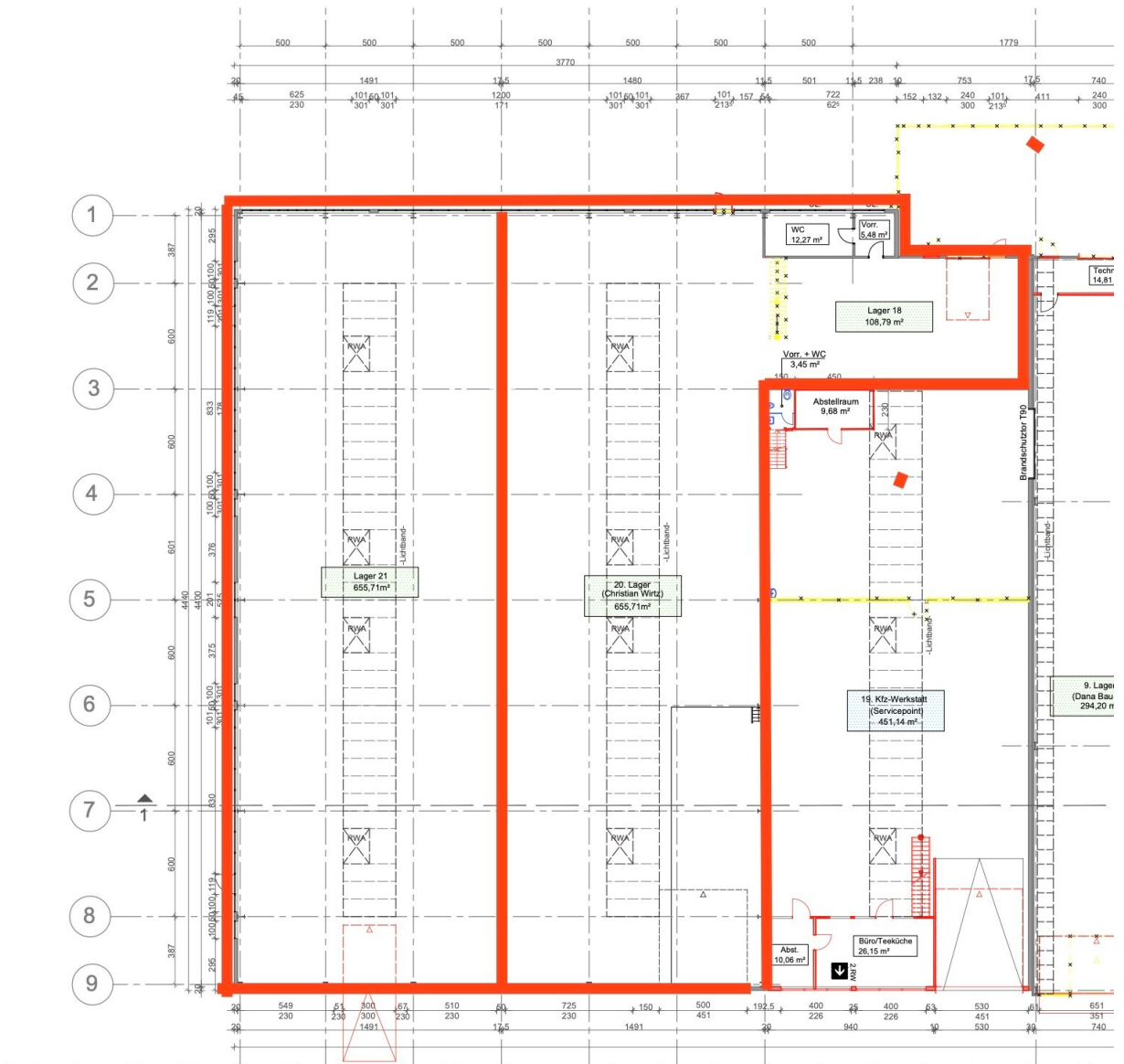
GR 2 Hallen
